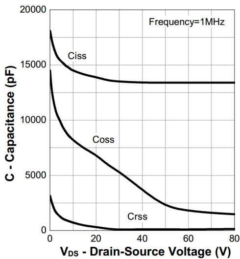
11. Capacitance
